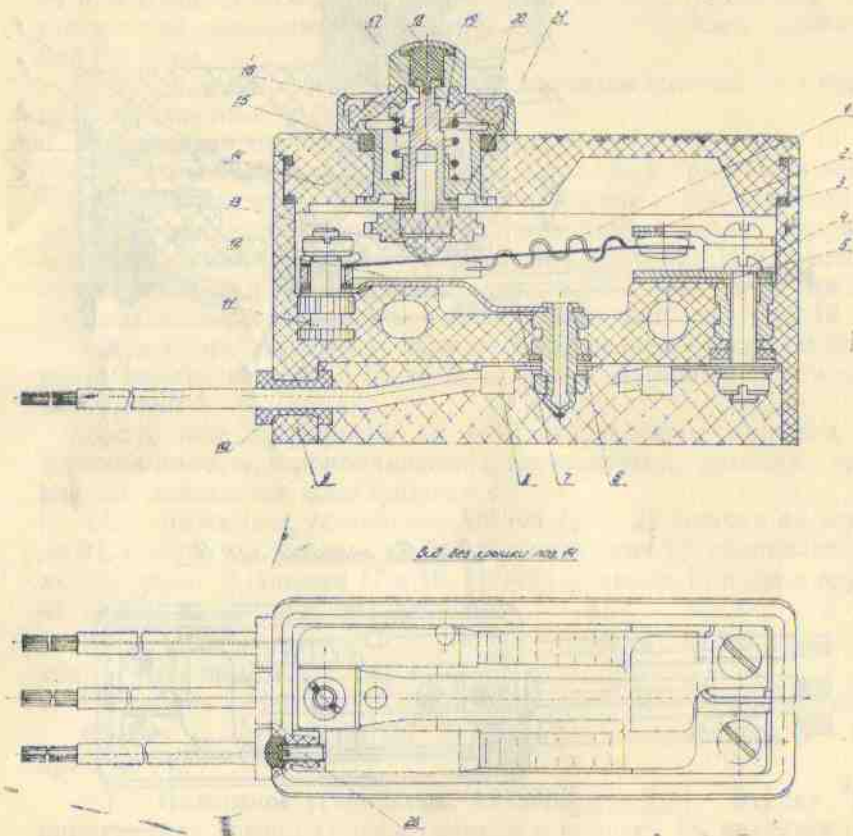
Рис. 2. Микровыключатель AM-800:
